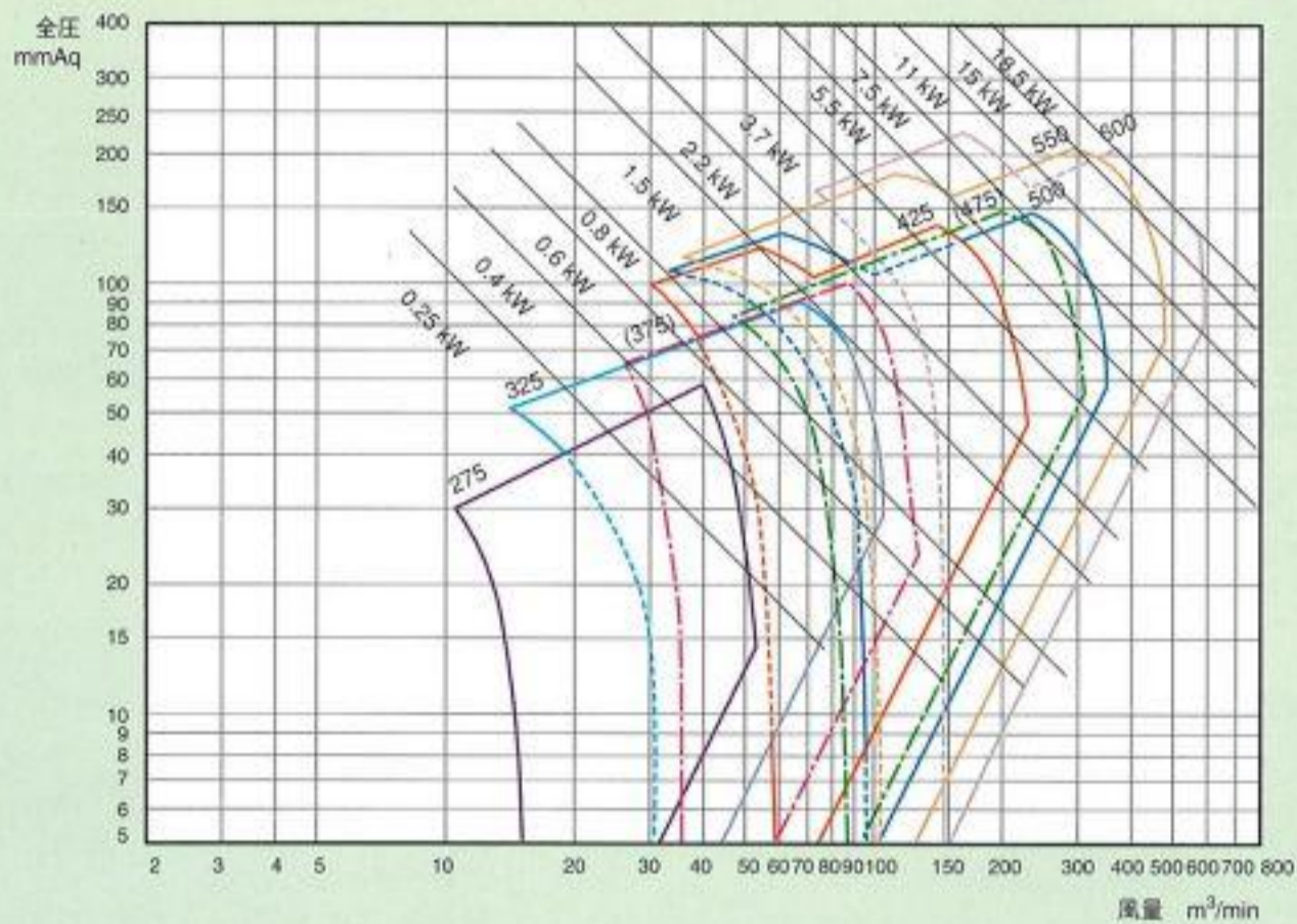
60Hz 2極選定表
