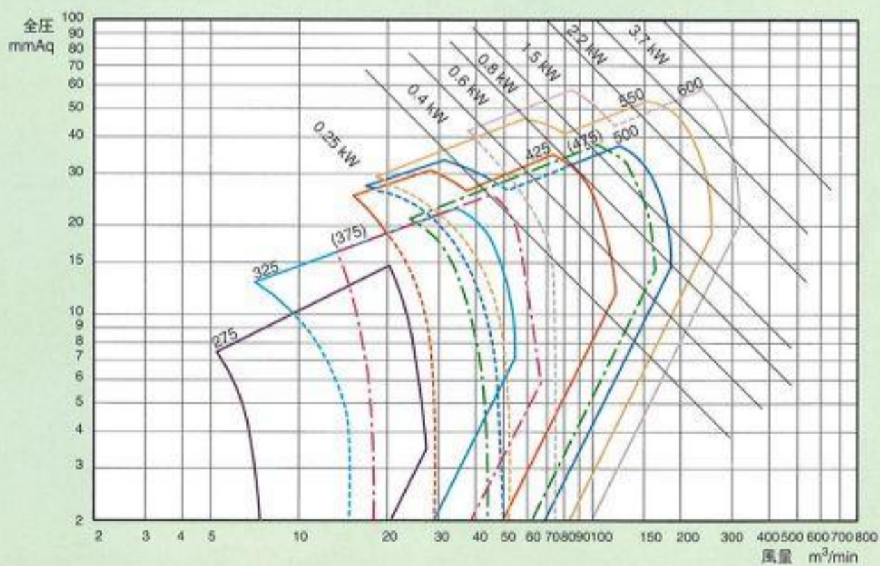
60Hz 4極選定表
